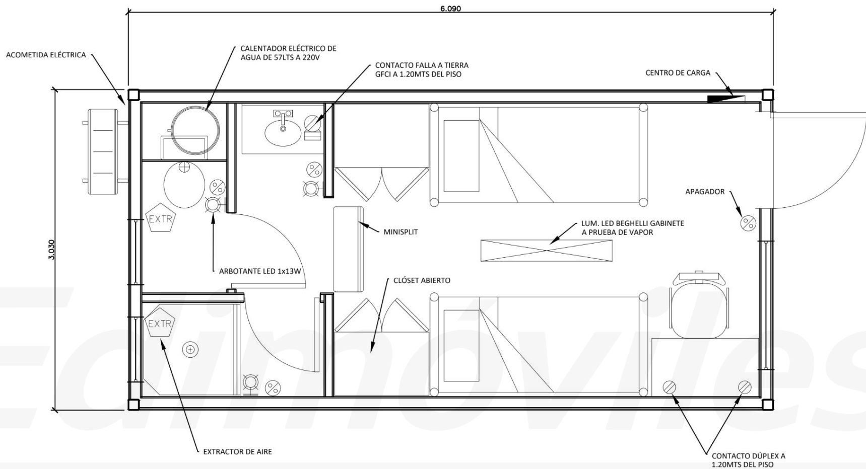
1 PLANTA TIPO 18.45M2
