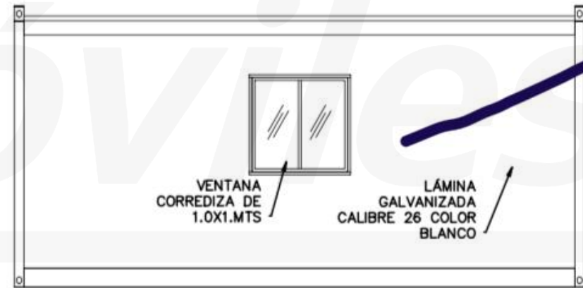
ALZADO POSTERIOR
