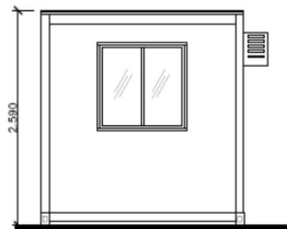
3 FACHADA LATERAL
