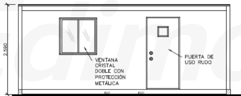
2 FACHADA DE ACCESO
