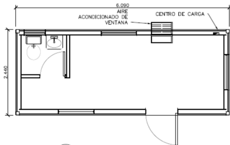
1 PLANTA ARQUITECTÓNICA
